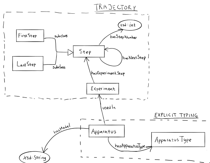
Fig. 12. Task B schema diagram.
